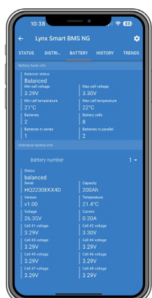
Vollständiger Überblick über alle Batteriedaten über VictronConnect (oder ein GX-Gerät und VRM)
